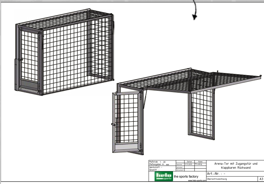
hochklappbarer Hinterbau am Fußballtor (Durchfahrtsmöglichkeit) Art.-Nr. 10-26
