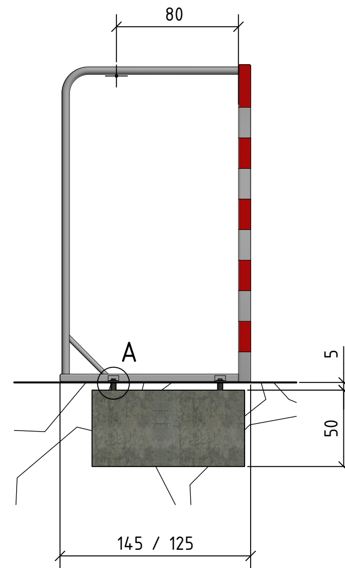
B ( 1 : 15 )
